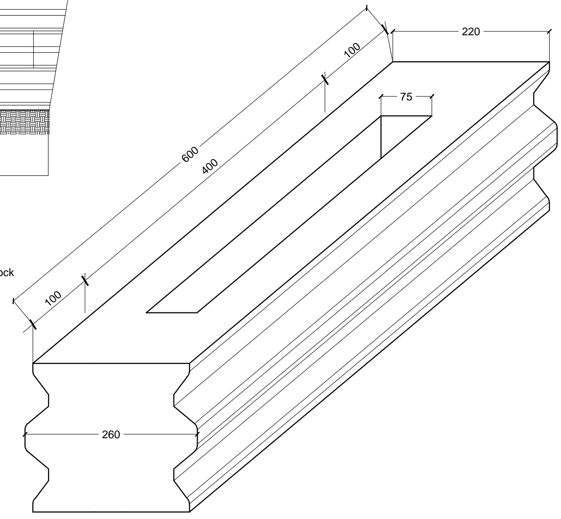
8c Axonometric INSET SCALE 1:5
